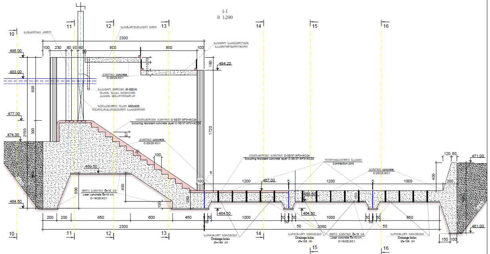
სურათი 4.2.1.1.2. ქსანი 1 ჰესის კაშხლის ჭრილი 1-1, მ 1:200
